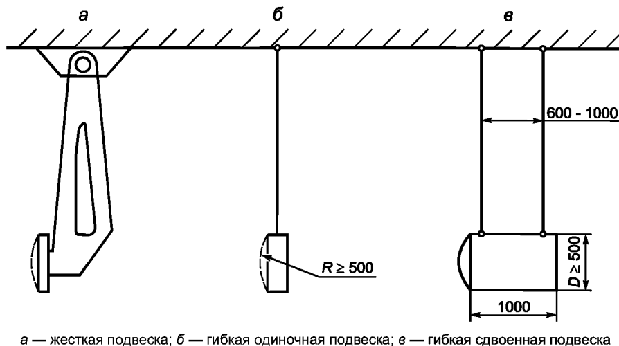
Рисунок 4 — Схема закрепления маятника
